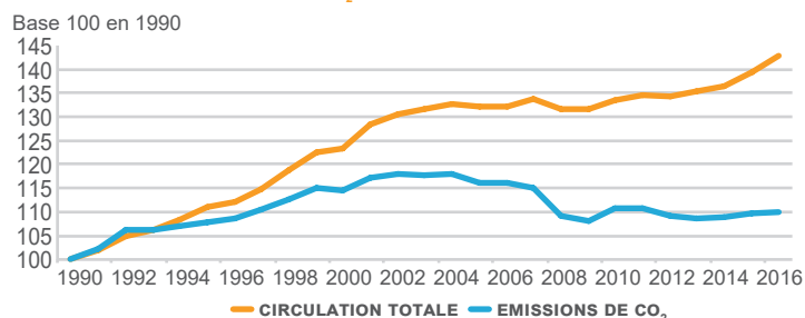
LA CIRCULATION DES VÉHICULES EN FRANCE ET LES ÉMISSIONS ASSOCIÉES DE CO 2 NETTES DES ÉNERGIES RENOUVELABLES
