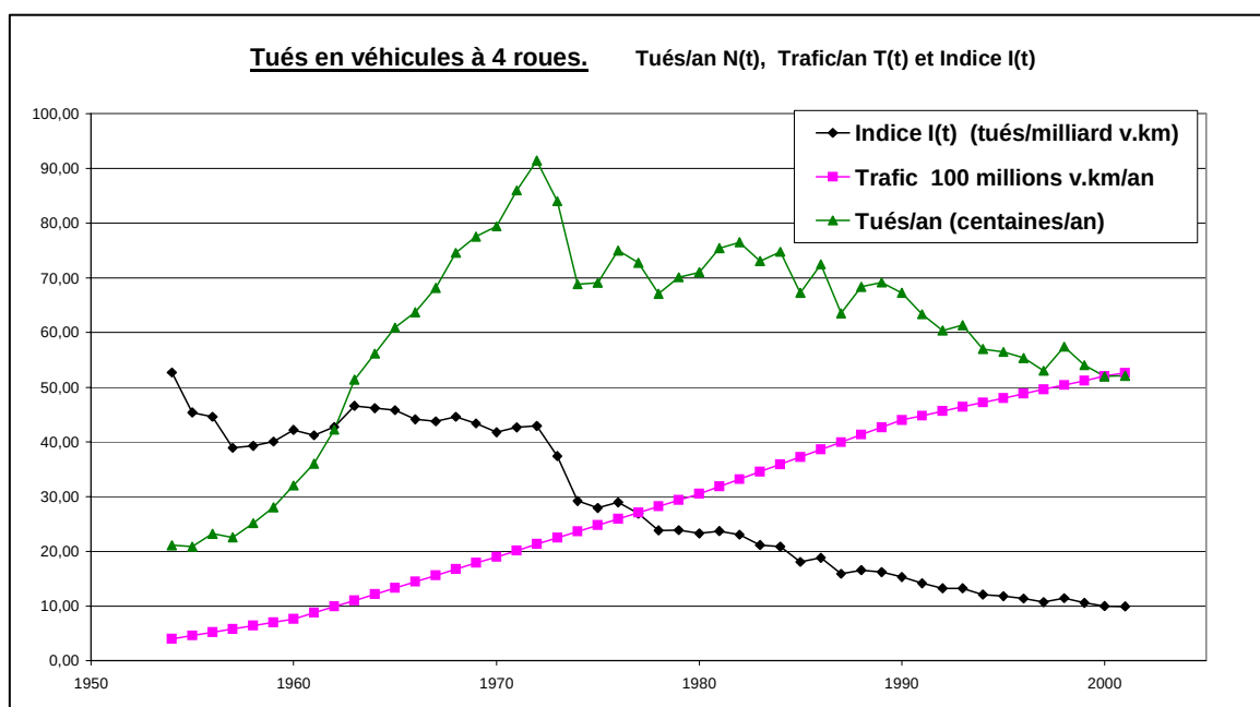
Figure 9. Évolution de N(t) , T(t) et I(t) pour les véhicules automobiles.
