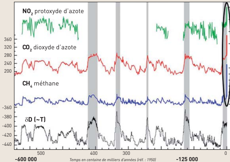
Figure 2. Variations de la température moyenne de la Terre et concentrations atmosphériques de quelques gaz à effet de serre, du quaternaire à nos jours. Reconstruction paléoclimatique sur la base de carottages glaciaires. Projet EPICA dome C.
