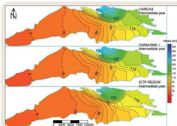
Figure 10. Cartes des niveaux piézométriques de la nappe de Quença-Silves pour trois scénarios distincts, obtenues selon la méthode de Penman-Grindley.
