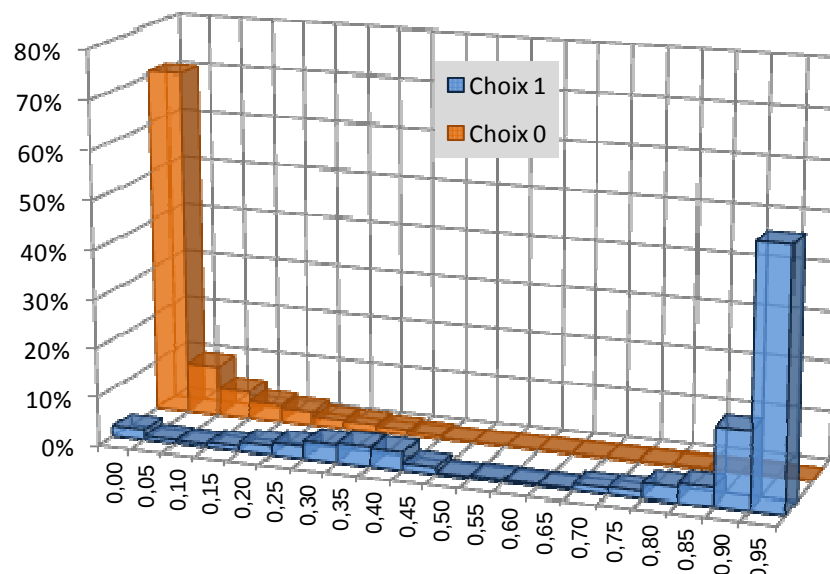
Figure 60 Modèle LOGIT multinomial - motif Santé - distribution des probabilités reconstituées pour les choix révélés (1) et pour les alternatives non choisies (0)
