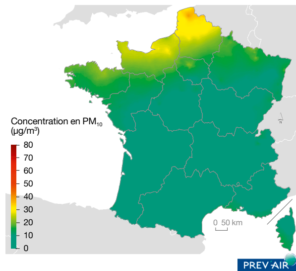
Carte 15 : moyennes des concentrations journalières de fond en PM_{10} , du 12 au 13 avril 2018
