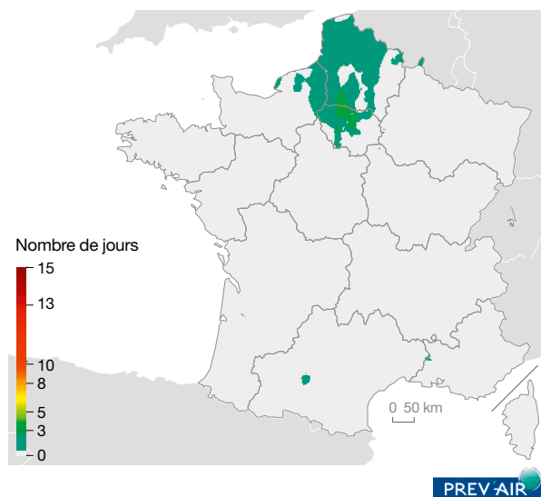
Carte 11 : nombre de jours de dépassement du seuil d'information pour l'ozone, entre le 23 et le 27 juillet 2018
