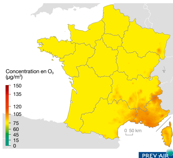
Carte 3 : moyenne des concentrations maximales journalières de fond en ozone, en 2018
