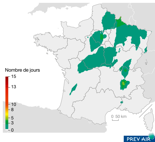
Carte 13 : nombre de jours de dépassement du seuil d'information pour l'ozone, entre le 2 et le 7 août 2018
