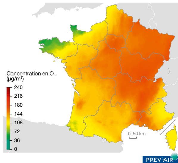
Carte 12 : moyenne des concentrations maximales journalières en ozone, du 2 au 7 août 2018
