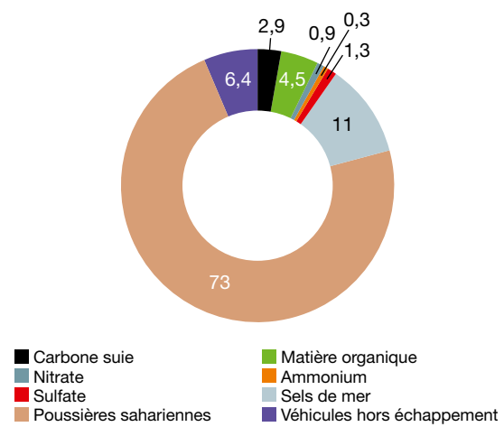
Graphique 6 : composition chimique des particules lors de l'épisode de pollution à Fort-de-France, en juin-juillet 2018 En %
