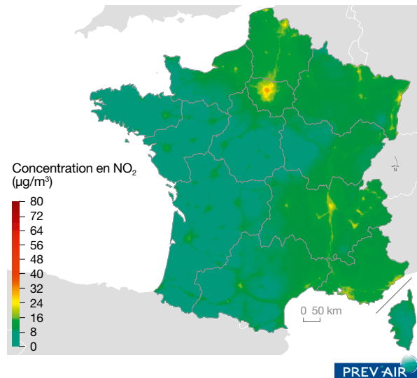
Carte 2 : concentrations moyennes annuelles de fond en \text{NO}_2 en France métropolitaine, en 2018
