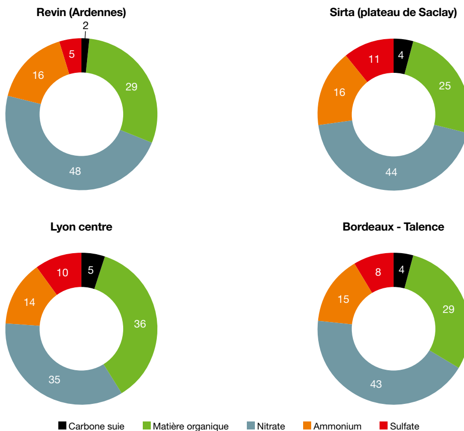
Graphique 5 : composition chimique des particules submicroniques, mesurée à l'aide d'analyseurs automatiques, le 21 février 2018
