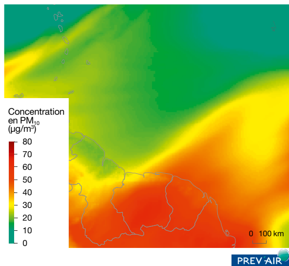
Carte 16 : concentrations moyennes journalières en PM 10 , le 30 mars 2018 en Guyane
