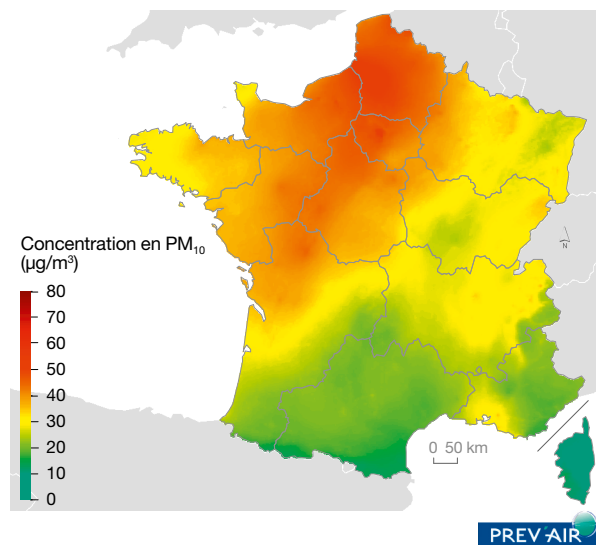
Carte 14 : moyennes des concentrations journalières de fond en PM_{10} , du 21 au 22 février 2018
