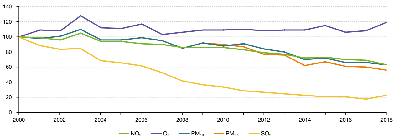
Graphique 2 : évolution des concentrations en SO 2 , NO 2 , O 3 , PM 10 et PM 2,5 en milieu urbain
