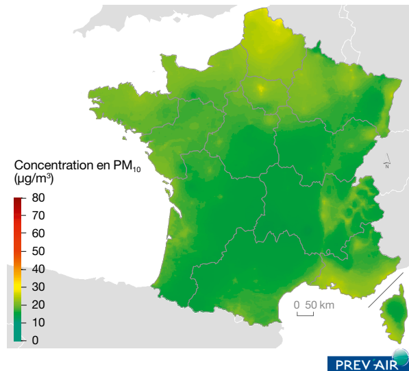
Carte 1 : concentrations moyennes annuelles de fond en \text{PM}_{10} en France métropolitaine, en 2018
