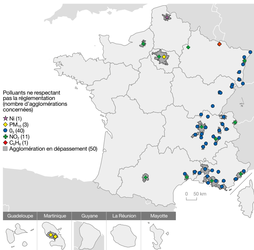
Carte 9 : agglomérations présentant en 2018 des dépassements des normes réglementaires pour la protection de la santé à long terme
