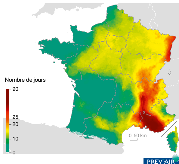
Carte 4 : nombre de jours pour lesquels la norme réglementaire pour la protection de la santé humaine à long terme pour l'ozone est dépassée en moyenne, sur la période 2016-2018
