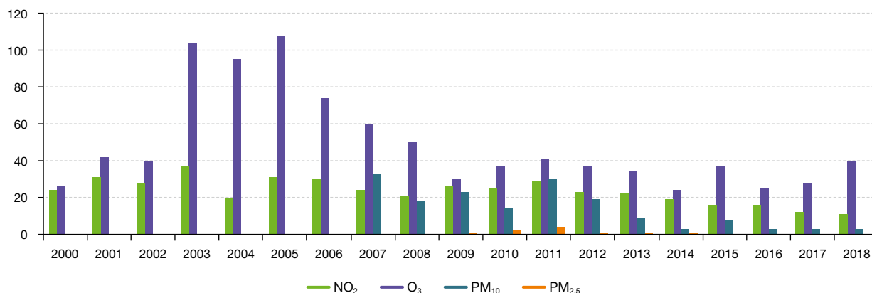
Graphique 4 : évolution des dépassements des normes réglementaires pour la protection de la santé à long terme dans les agglomérations pour les polluants les plus problématiques
