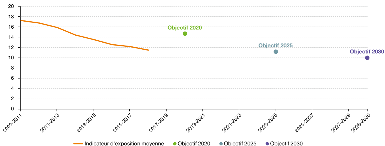
Graphique 3 : évolution de l'indicateur d'exposition moyenne aux \text{PM}_{2,5} en fond urbain
