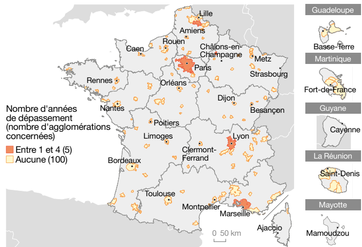
Carte 8 : PM 2,5 (période 2009-2018)
