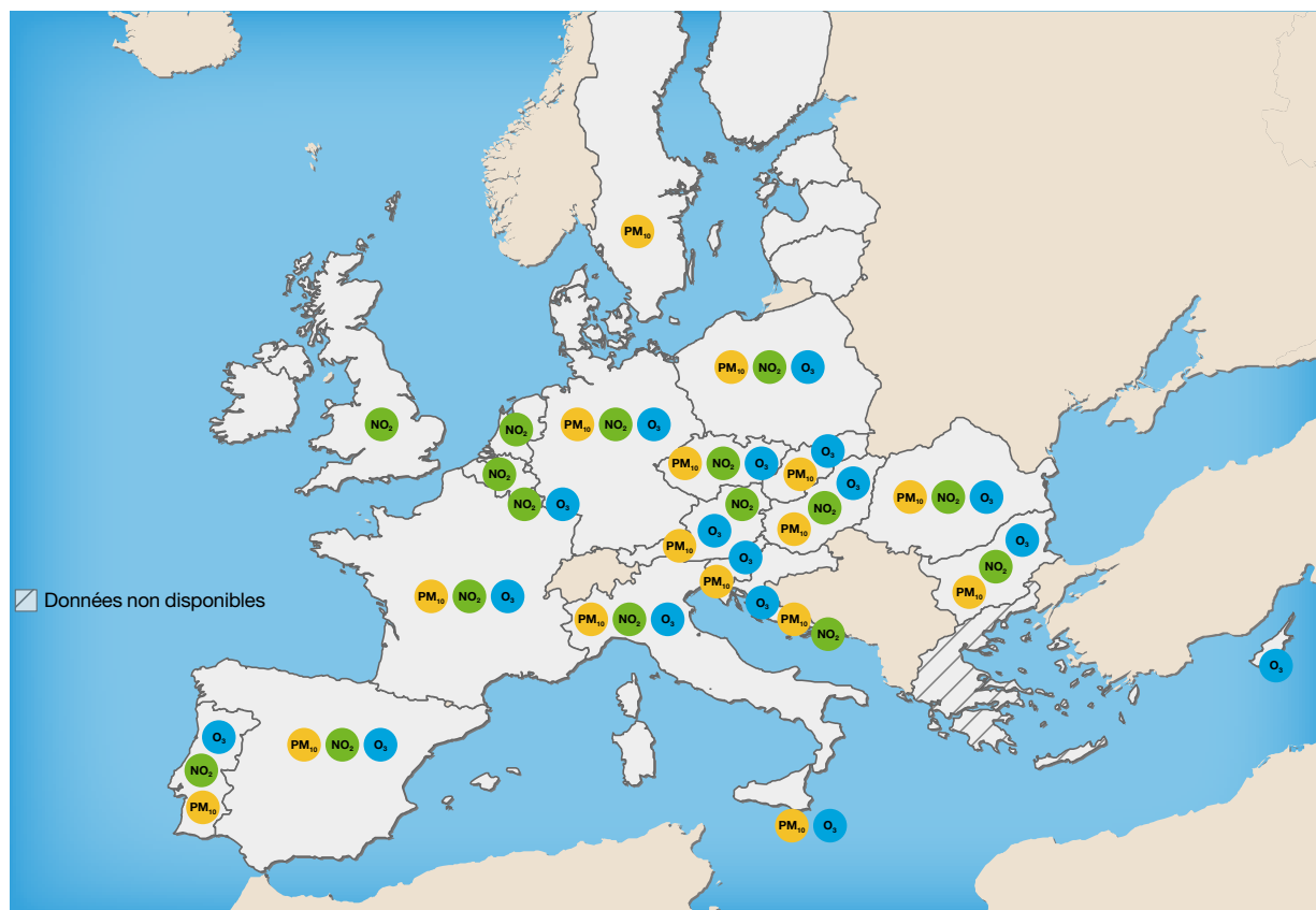
Carte 17 : dépassements des normes réglementaires de qualité de l'air pour la protection de la santé à long terme dans l'UE28, en 2017
