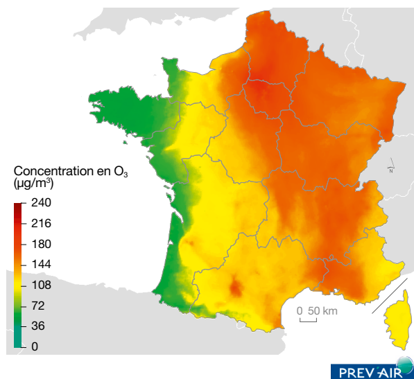
Carte 10 : moyenne des concentrations maximales journalières en ozone, du 23 au 27 juillet 2018
