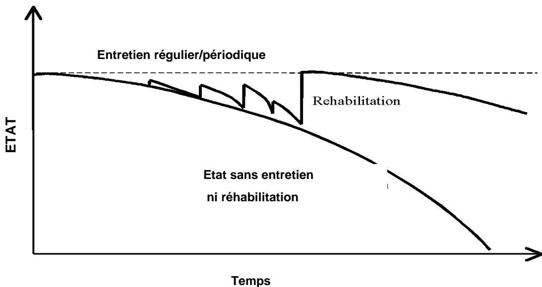
Détérioration d'une route et résultat de l'entretien
