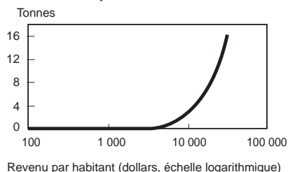
Emissions moyennes de gaz carbonique par habitant a
