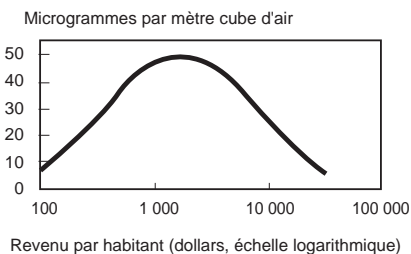
Concentrations moyennes de dioxyde de soufre dans les villes
