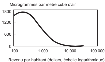
Concentrations moyennes de particules dans les villes
