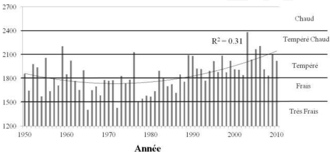
Figure 7 : Evolution de l'indice de Huglin (IH) à Saumur, de 1950 à 2010. (Source des données : Météo-France). (Neethling et al, 2012)
