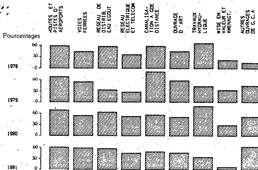
Graphique 4 PART DES TRAVAUX D'AMÉLIORATION-ENTRETIEN DU GÉNIE CIVIL ET AGRICOLE RÉALISÉS PAR LES ENTREPRISES DE 200 SALARIÉS ET PLUS DE 1978 A 1981 SELON LA NATURE DE L'OUVRAGE
