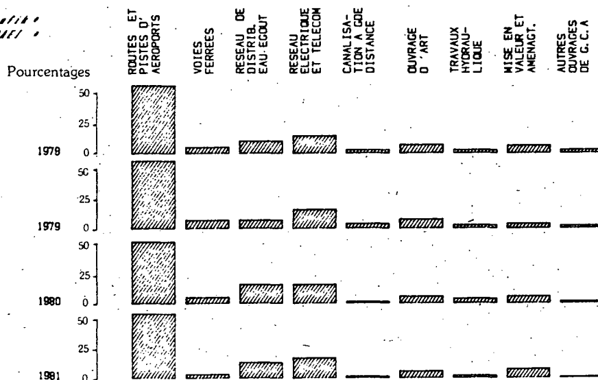
Graphique 4 PART DES TRAVAUX D'AMÉLIORATION-ENTRETIEN DU GÉNIE CIVIL ET AGRICOLE RÉALISÉS PAR LES ENTREPRISES DE 200 SALARIÉS ET PLUS DE 1978 A 1981 SELON LA NATURE DE L'OUVRAGE
