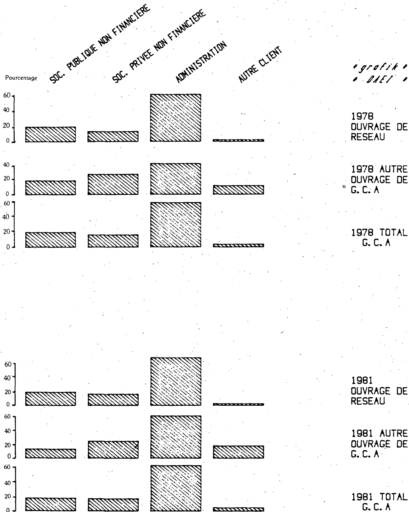
Graphique 9 TRAVAUX D'AMÉLIORATION-ENTRETIEN SELON LA NATURE DE L'OUVRAGE ET LE CLIENT EN 1978 ET 1981 (en %)
