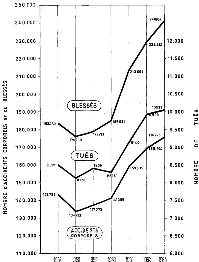
Fig. 2. — Accidents corporels et victimes de 1957 à 1963.
