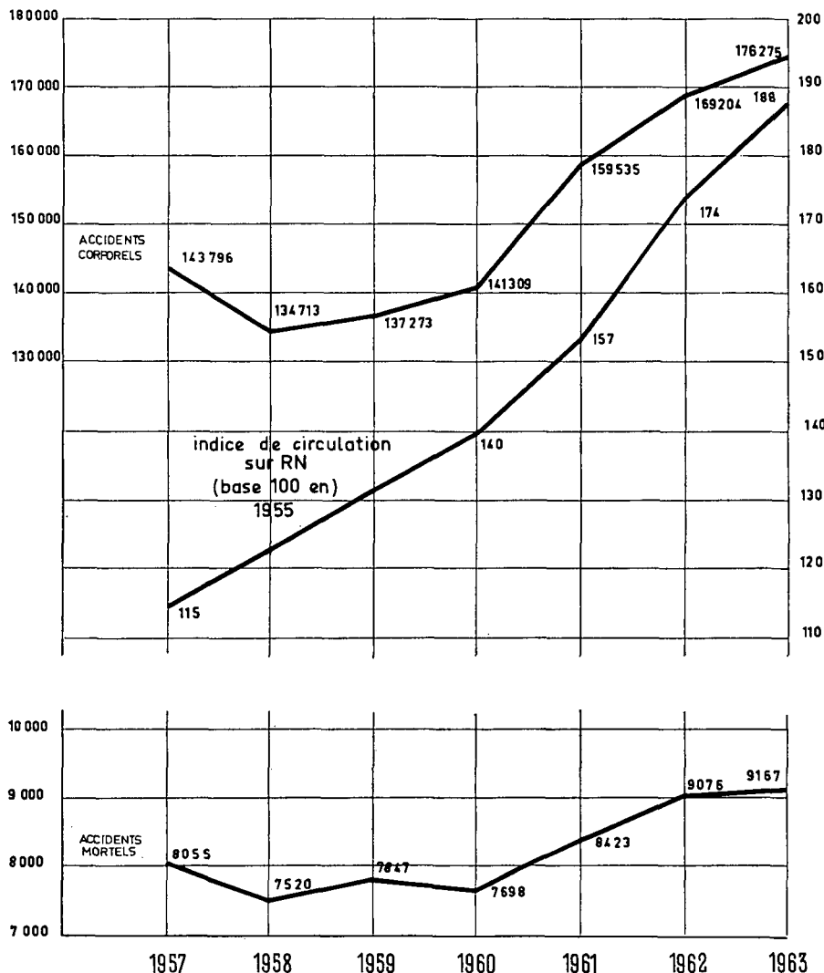
Fig. 3. — Accidents et circulation de 1957 à 1963.
