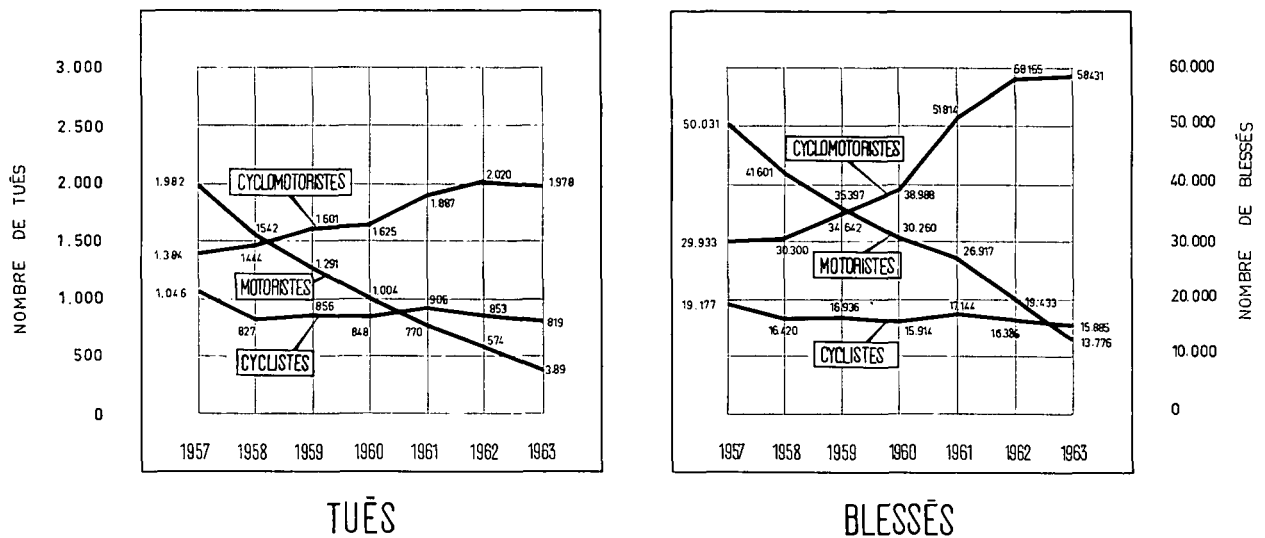
Fig. 7. — Victimes sur « deux roues » de 1957 à 1963.
