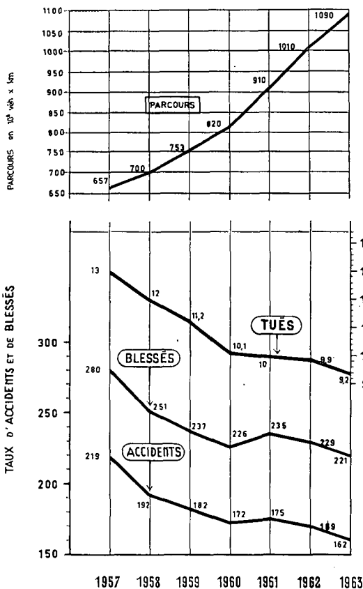
Fig. 1. — Taux par unité de parcours (10 8 véh × km) de 1957 à 1963.
