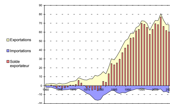
Fig. 5 : Commerce extérieur d'électricité depuis 1960 (en TWh).
