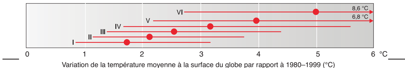
Figure RiD.8. Valeurs estimées du réchauffement à long terme (sur plusieurs siècles) correspondant aux six catégories de scénarios de stabilisation élaborés par le Groupe de travail III pour le quatrième Rapport d'évaluation (tableau RiD.6). L'échelle des températures a été décalée de - 0,5 °C par rapport au tableau RiD.6, afin de tenir compte du réchauffement intervenu entre l'époque préindustrielle et 1980-1999. La température moyenne à la surface du globe approche de l'équilibre au bout de quelques siècles pour la plupart des niveaux de stabilisation. Selon les scénarios d'émissions de GES qui entraînent, d'ici à 2100, une stabilisation à des niveaux comparables à ceux des scénarios B1 et A1B du SRES (600 et 850 ppm équiv.-CO 2 , catégories IV et V), les modèles indiquent que la hausse de la température mondiale à l'équilibre serait réalisée dans une proportion de 65 à 70 % environ au moment de la stabilisation, en fixant la sensibilité du climat à 3 °C. La température à l'équilibre pourrait être atteinte plus tôt avec les scénarios de stabilisation à des niveaux nettement inférieurs (catégories I et II, figure RiD.11). (Figure 3.4)
