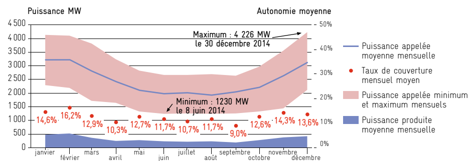
Puissance électrique appelée et produite mensuellement en 2014
