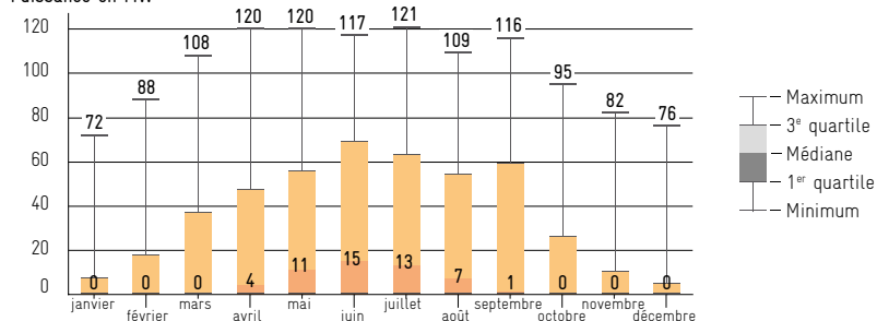
Evolution mensuelle du maximum, du minimum et de la médiane de production mensuelle photovoltaïque en 2014
