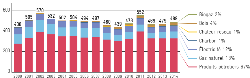
Consommation de l'agriculture corrigée du climat
