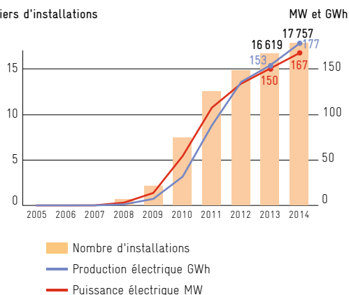
Nombre, puissance et production des installations solaires photovoltaïques
