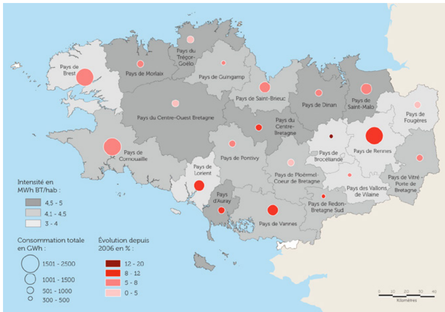
Consommation d'électricité par pays sur le réseau de distribution en 2014
