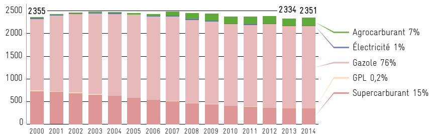
Consommation du transport corrigée du climat
