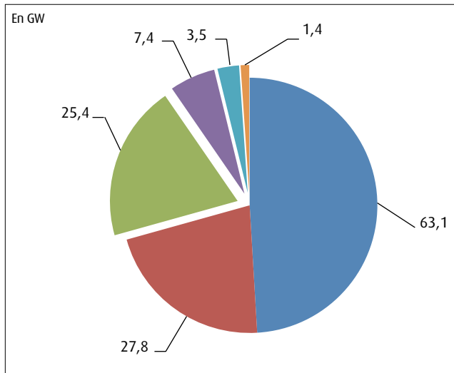
Puissance installée au 31/12/2012 par filières Total 128,7 GW
