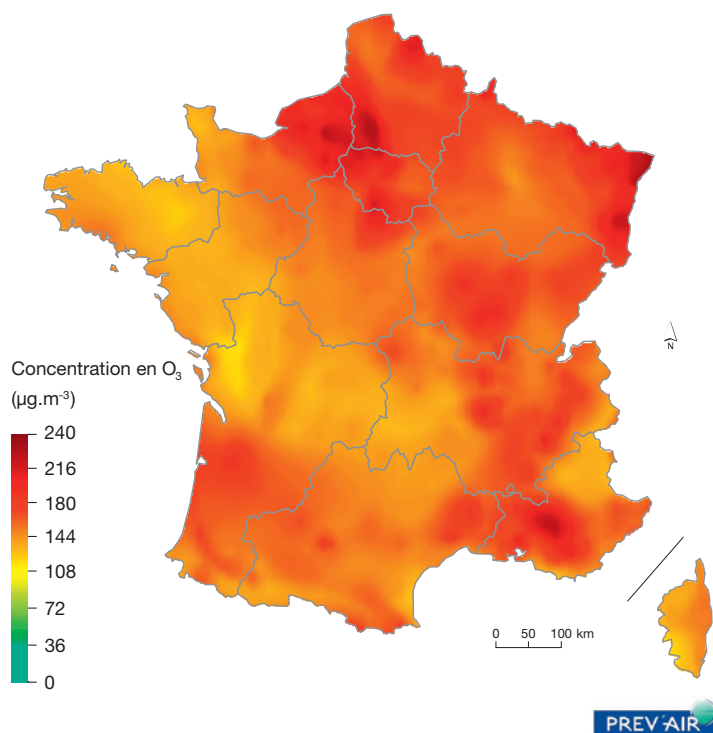
Carte 3 : concentrations maximales horaires de fond en \text{O}_3 du 30 juin au 7 juillet 2015
